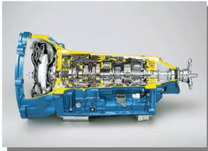
自動車のミッションケース
